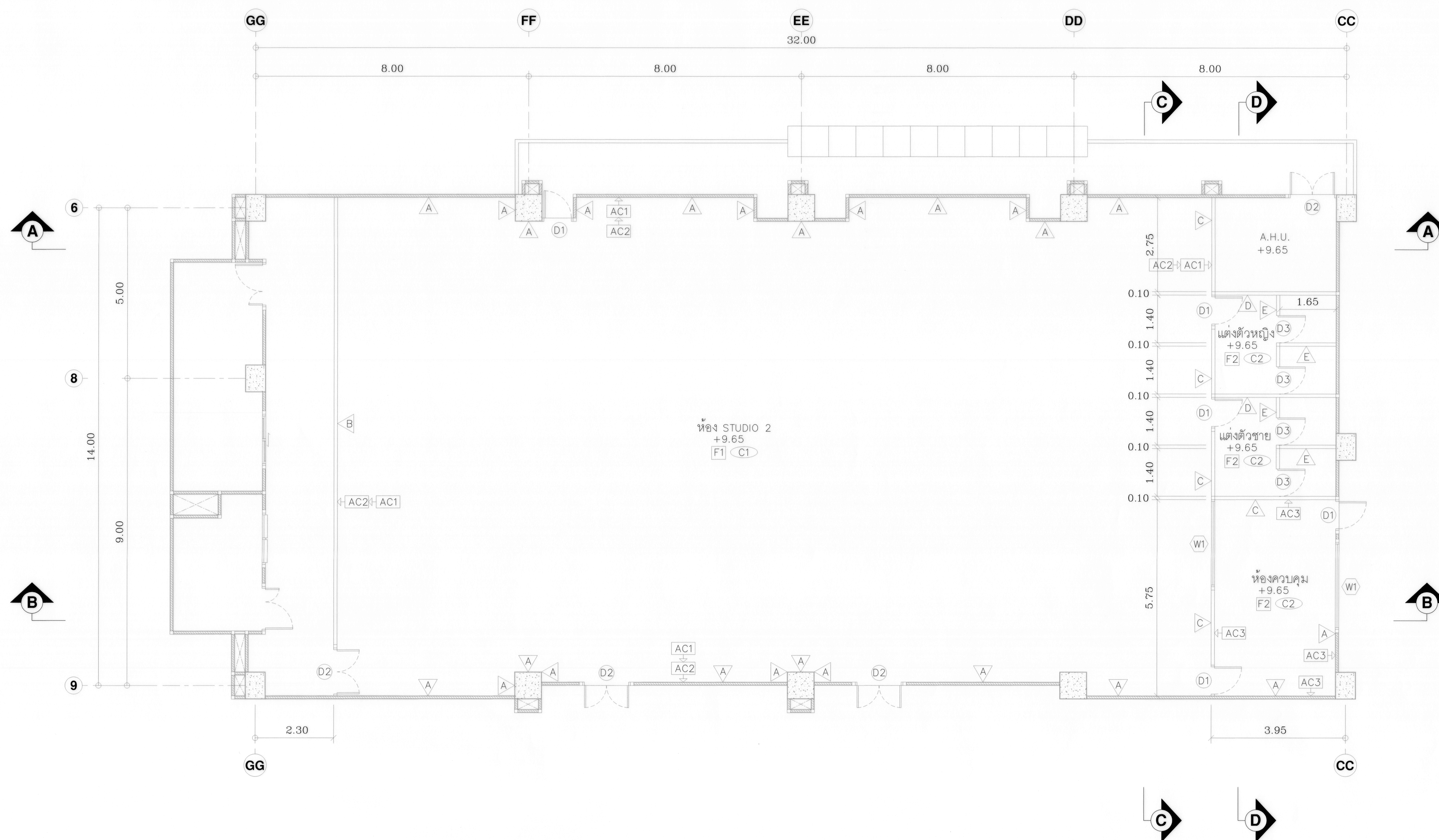
แปลนห้อง STUDIO 2 (ปรับปรุง) SCALE 1 : 50
